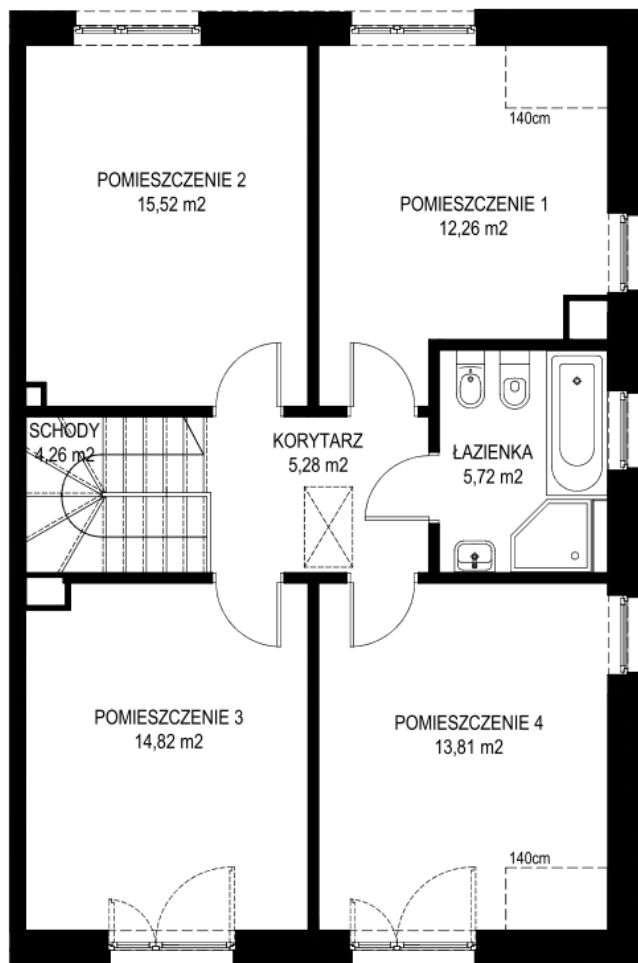
RZUT PODDASZA
